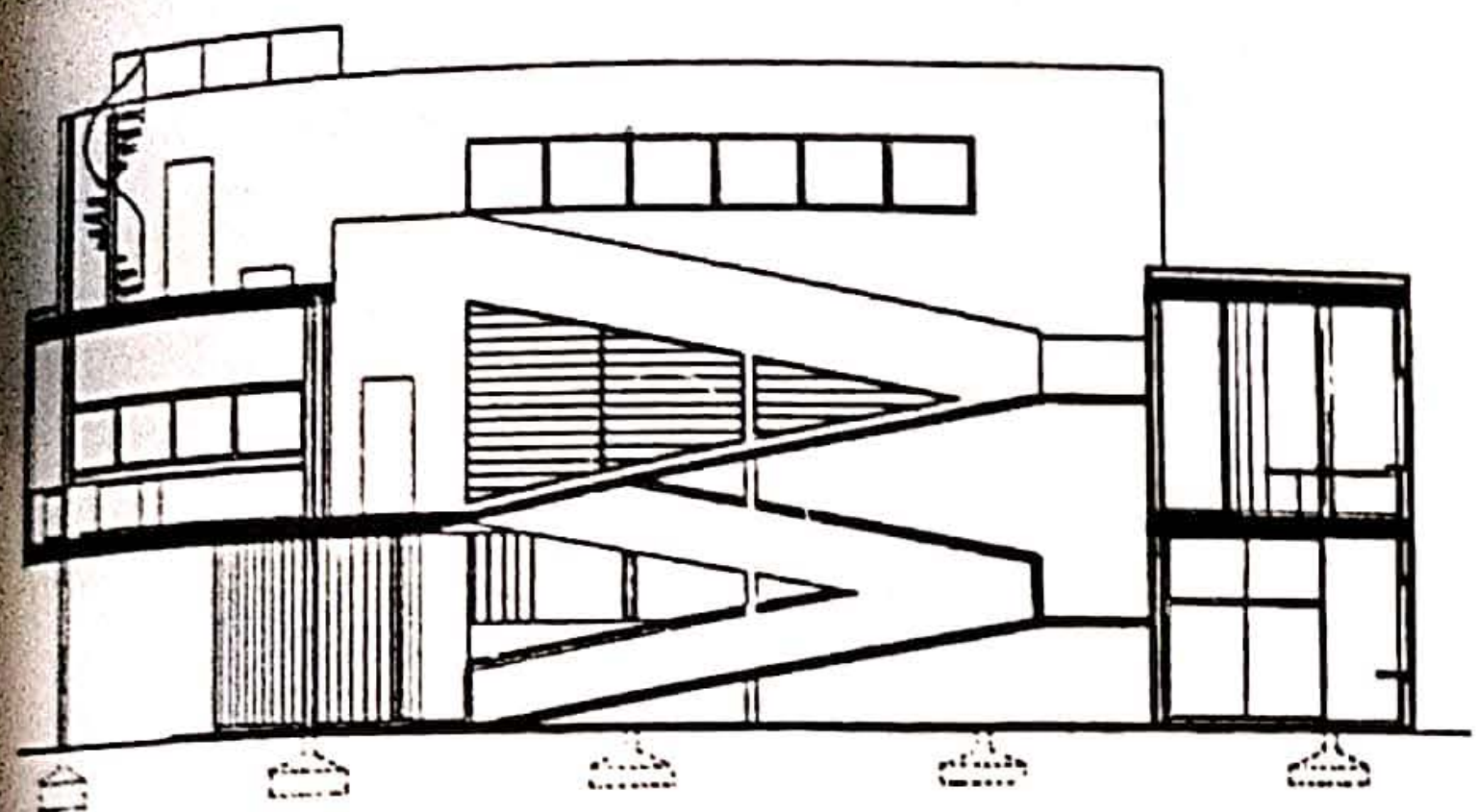
Coupe en travers Cross section Querschnitt
